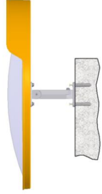
2-DUVARA MONTAJ ŞEKLİ
